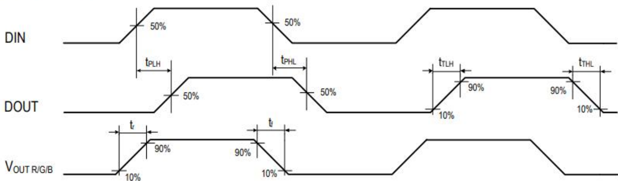
Fig.动态参数测试示意图
