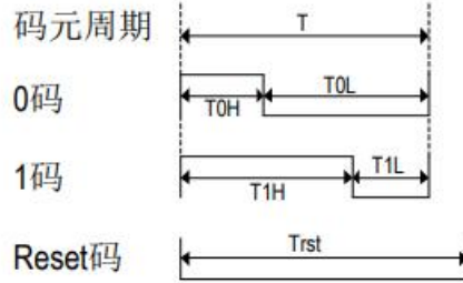
Fig. 归零码数据通信协议图
