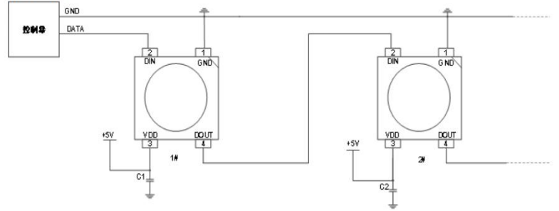
Fig. 产品应用示意图
