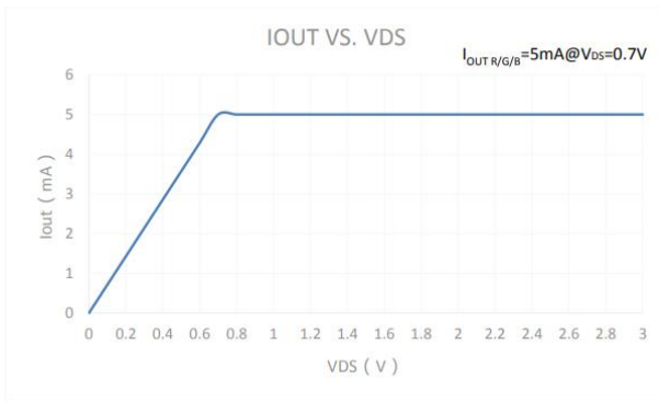
Fig. I OUT 与 OUTR/G/B 端口电压 V_{DS} 的关系图
